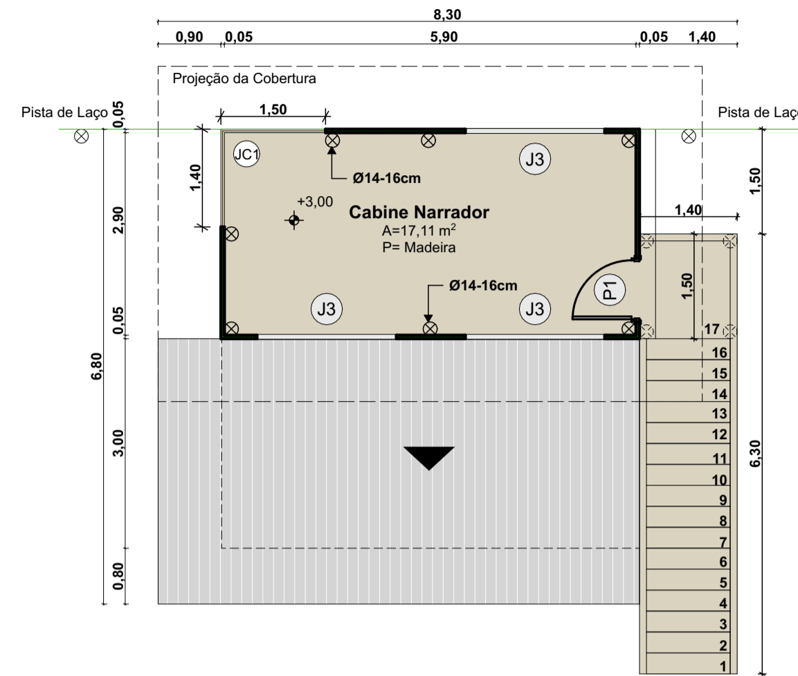
PLANTA SUPERIOR CABINE INSCRIÇÃO/ NARRADOR ÁREA TERREO: 44,82m² ÁREA 2ª PAV.: 18,00m² ÁREA TOTAL: 62,82 ESC: 1/75
