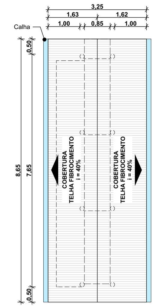
COBERTURA BRETE DE SAÍDA ESC: 1/75
