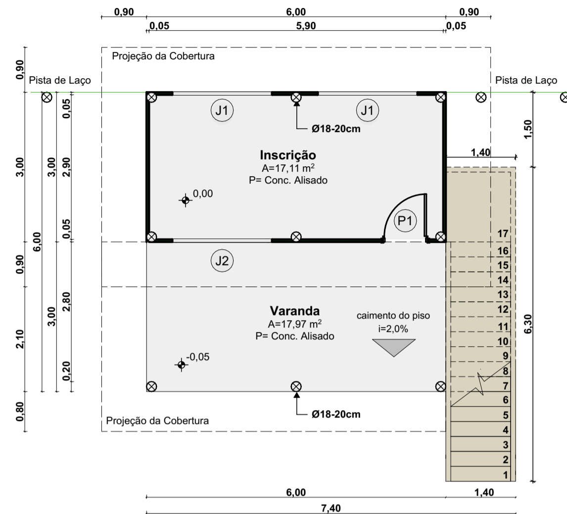
PLANTA BAIXA CABINE INSCRIÇÃO/ NARRADOR ÁREA TERREO: 44,82m² ÁREA 2ª PAV.: 18,00m² ÁREA TOTAL: 62,82 ESC: 1/75
