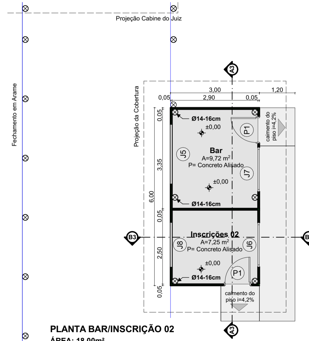
COBERTURA BAR/ INSCRIÇÕES 02 ESC: 1/75
